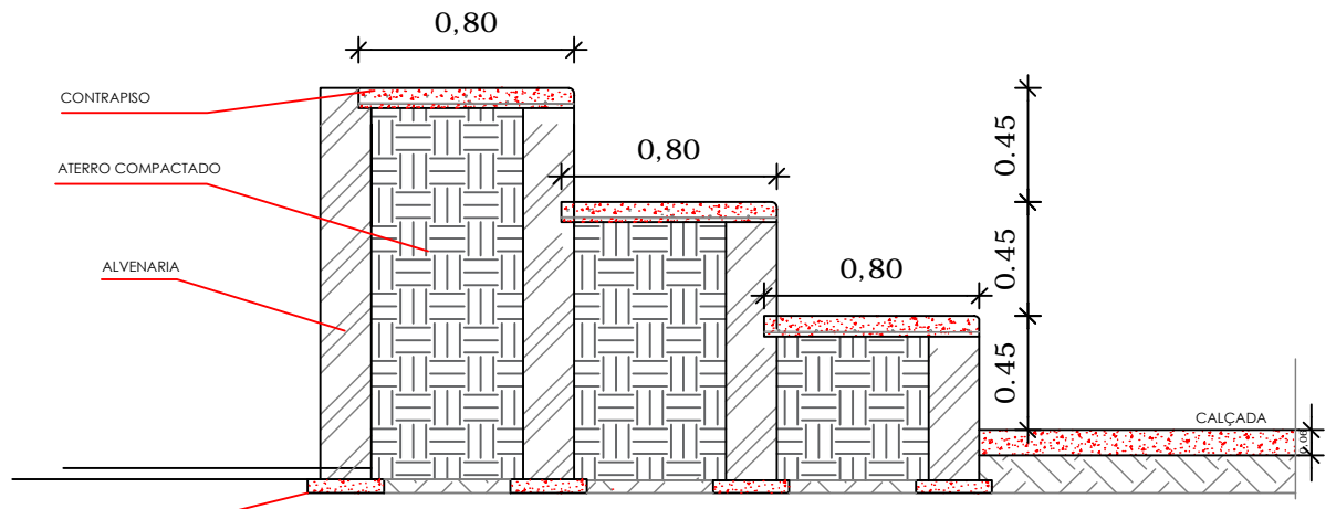
DETALHE DA ARQUIBANCADA ESCALA 1:20
