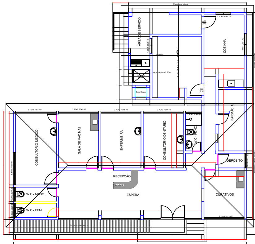
PLANTA BAIXA
