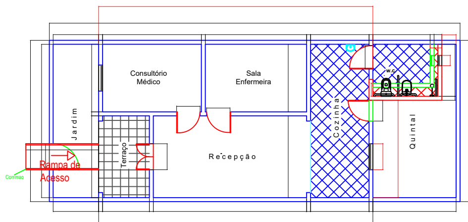
Planta Baixa
