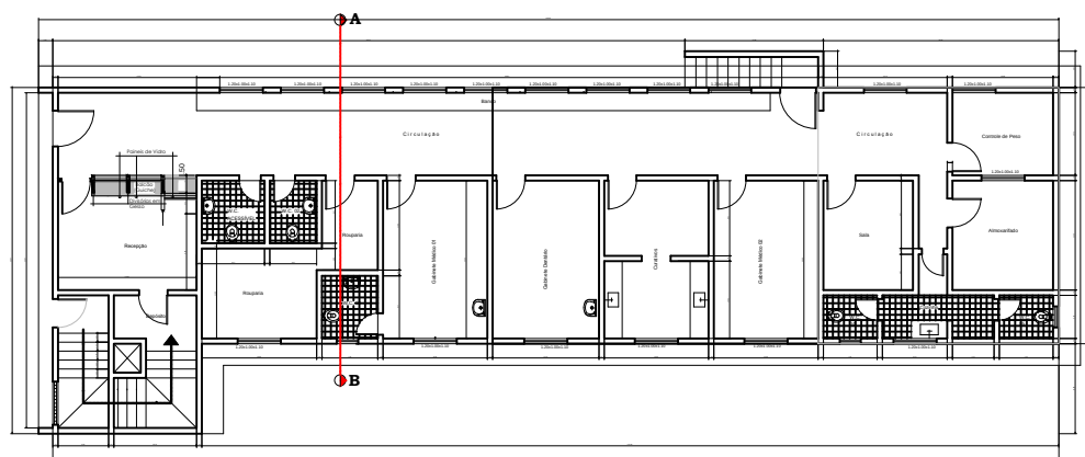
Planta Baixa - Pav. Térreo ESCALA - 1/100
