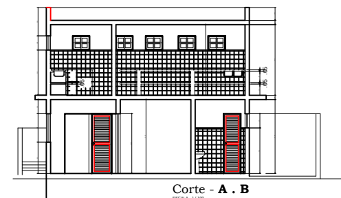
Corte - A . B ESCALA - 1/100
